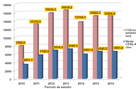
Figura 20: Suma de indicadores de la generación bruta, combustible sustituido y CO2 no generado.
