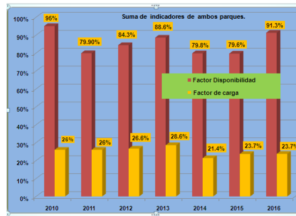
Figura 17: Relación del factor de disponibilidad y capacidad.
