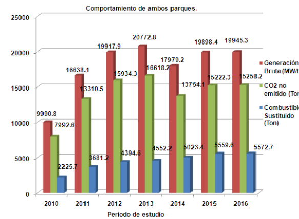
Figura 18: Relación entre generación bruta, combustible sustituido y CO2 no generado.
