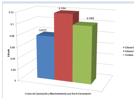
Figura 26: Costos de operación y mantenimiento por generación de Mw/h.
