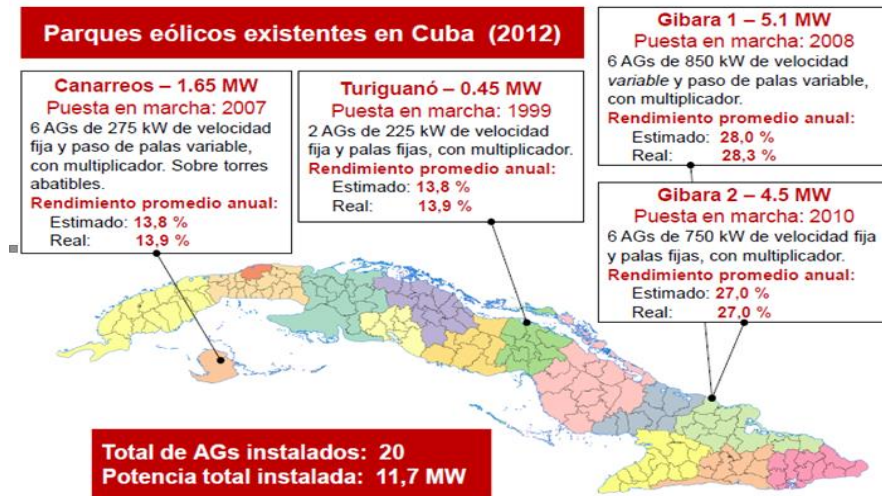
Figura 10: Parques eolicos existentes en Cuba.
