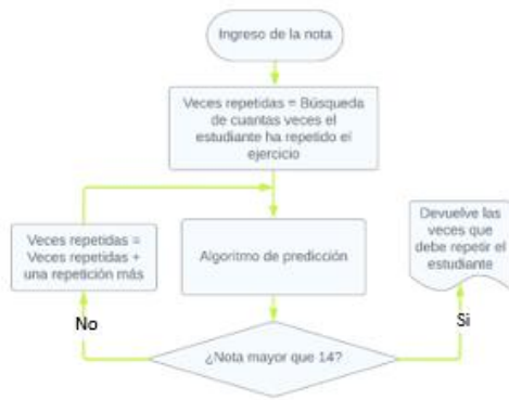
Fig. 5: Diagrama de flujo para predecir cuantas veces debe repetir un ejercicio el estudiante.
