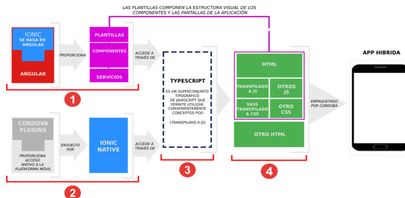
Fig. 9: Esquema del desarrollo de una aplicación móvil en Ionic Angular.
