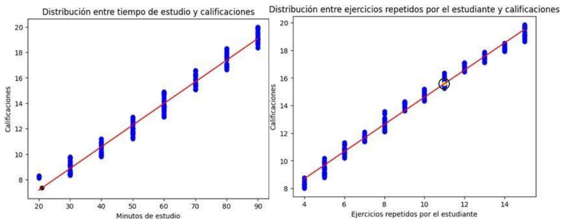
Fig. 3: Grafico de dispersión de datos de calificaciones y tiempo. Fig. 4: Grafico de dispersión de datos de calificaciones y ejercicios repetidos por el estudiante.
