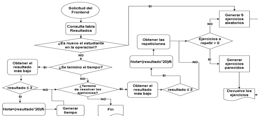
Fig. 7: Diagrama de flujo de la función de los algoritmos inteligentes.
