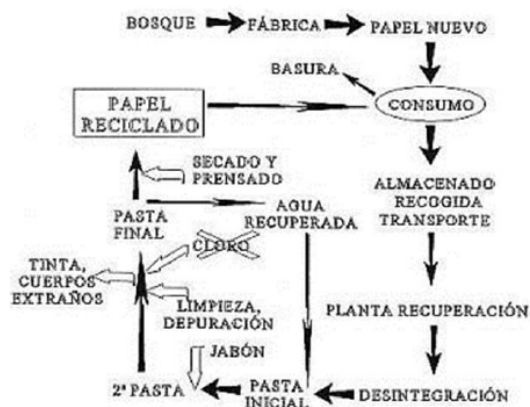
Figura 1. Esquema del proceso de fabricación del papel reciclado. Fuente: (Cadme & Miranda, 2012)
